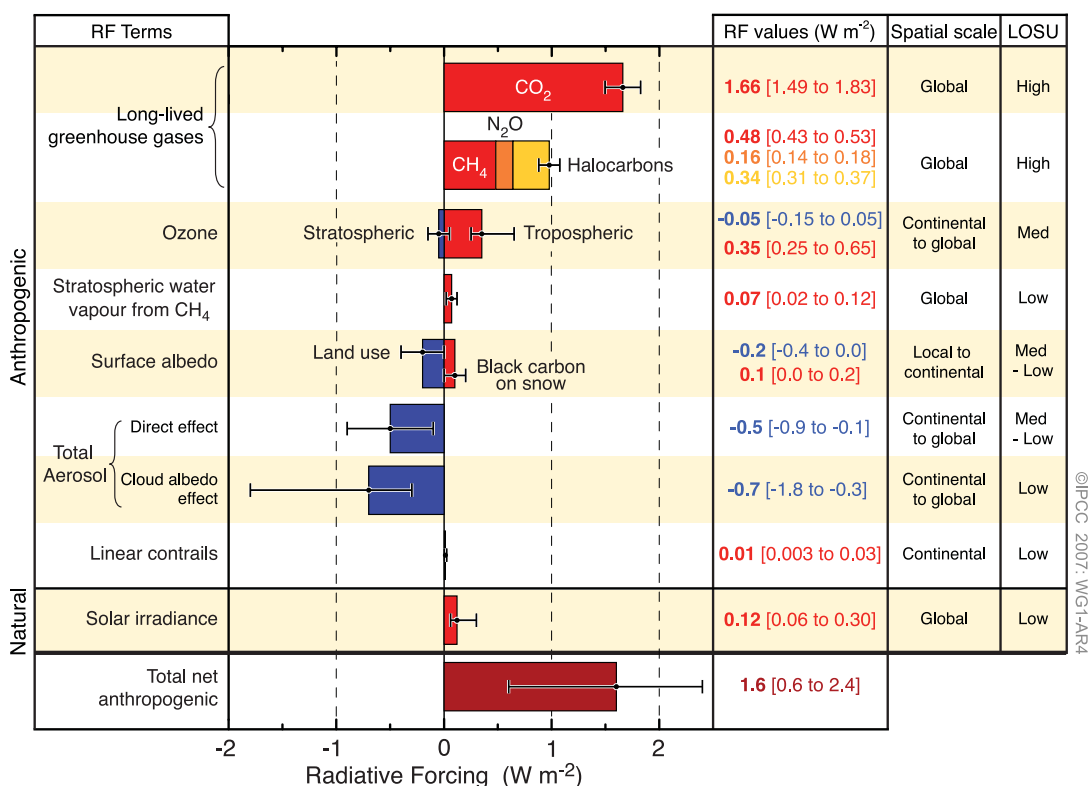
Рис. SPM-2. Компоненти випромінювальних потужностей
