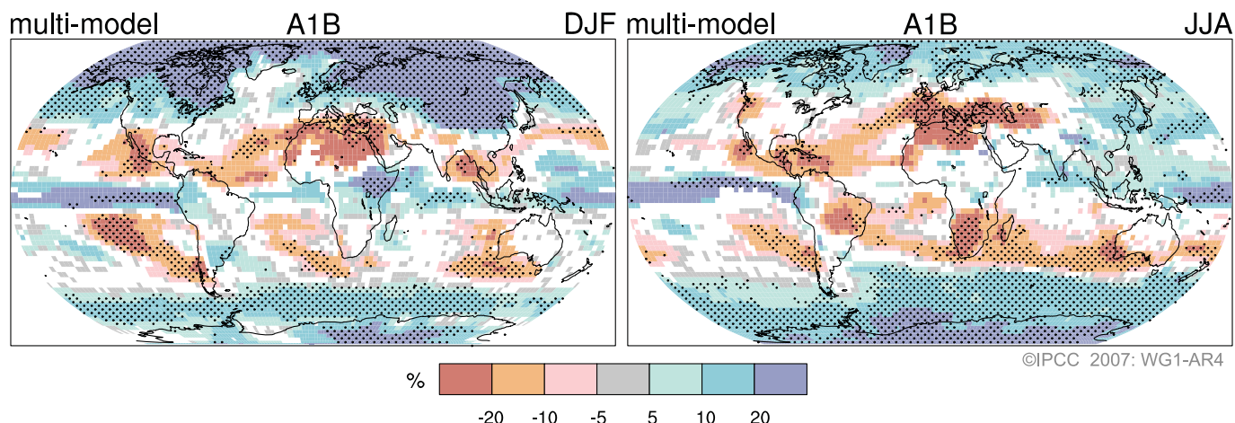
Рис. SPM-7. Відносні зміни опадів (у %) на період 2090–2099 рр. відносно 1980–1999 рр. Дані є багатомодельними середніми величинами, що базуються на сценарії SRES A1B для грудня – лютого (зліва) та червня–серпня (справа). Білі зони означають регіони, для яких менше 66% моделей дають подібні результати змін, а заштриховані зони – більше 90% моделей співпадають у прогнозах змін. {Рис. 10.9}
