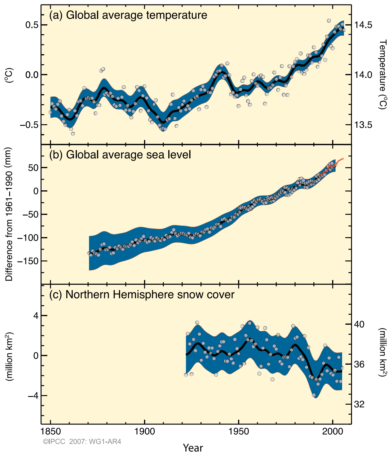
Рис. SPM-3. Зміни температури, рівня моря та снігового покриву північної півкулі
