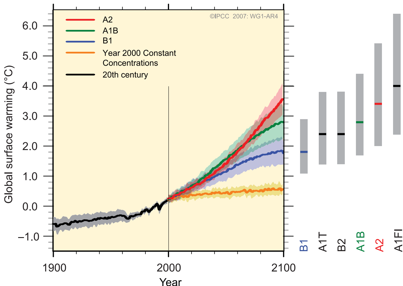
Рис. SPM-5. Суцільні лінії позначають багатомодельні середні глобальні показники потепління поверхні суші (у порівнянні з 1980 – 1999 рр.) для сценаріїв A2, A1B і B1, показані як продовження XX ст. Затінені зони показують межі \pm 1 стандартного відхилення щорічних середніх даних за окремими моделями. Помаранчевою лінією позначені дані експерименту, коли концентрації утримувались стабільними на рівні 2000 р. Сірі стовпці праворуч з суцільною лінією всередині стовпця показують найвірогідніші зміни та ймовірні відхилення, визначені для шести маркерних сценаріїв SRES. Визначення найвірогідніших змін та ймовірних відхилень включає AOGCMs, подані на лівій стороні рисунку, а також результати ієрархії незалежних моделей обмежень для спостережень {Рис. 10.4 та 10.29}
